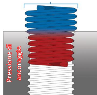
Diametro allo stato libero
